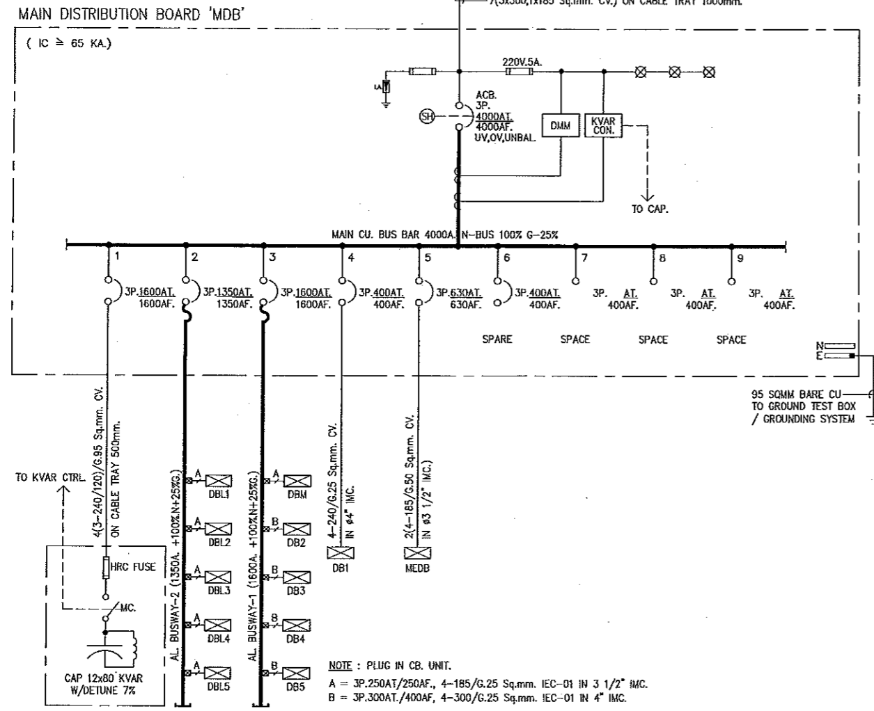
ไดอะแกรมระบบไฟฟ้า 1
