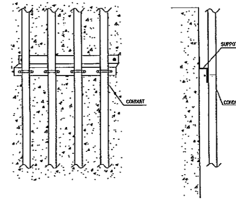
แบบตัวอย่างติดตั้งท่อโรยหรือร่นผนัง
