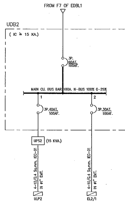
ไดอะแกรมระบบไฟฟ้า 2
