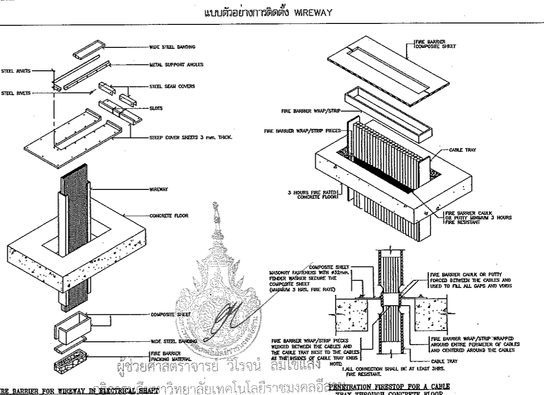
แบบตัวอย่างการติดตั้ง WAREWAY แบบตัวอย่างการติดตั้ง FIRESTOP
