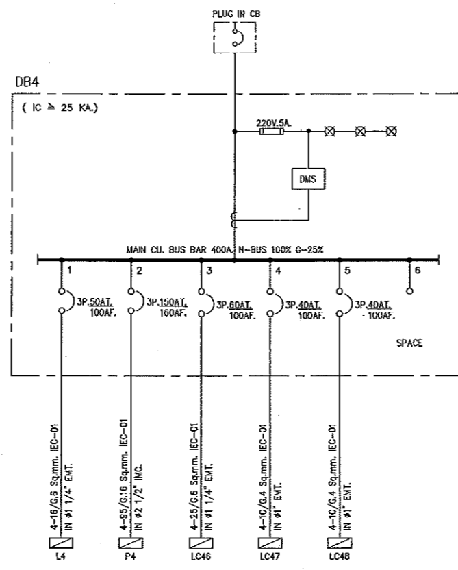
ไดอะแกรมระบบไฟฟ้า 3
