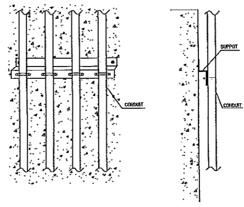
แบบตัวอย่างติดตั้งท่อร้อยสายผนัง
