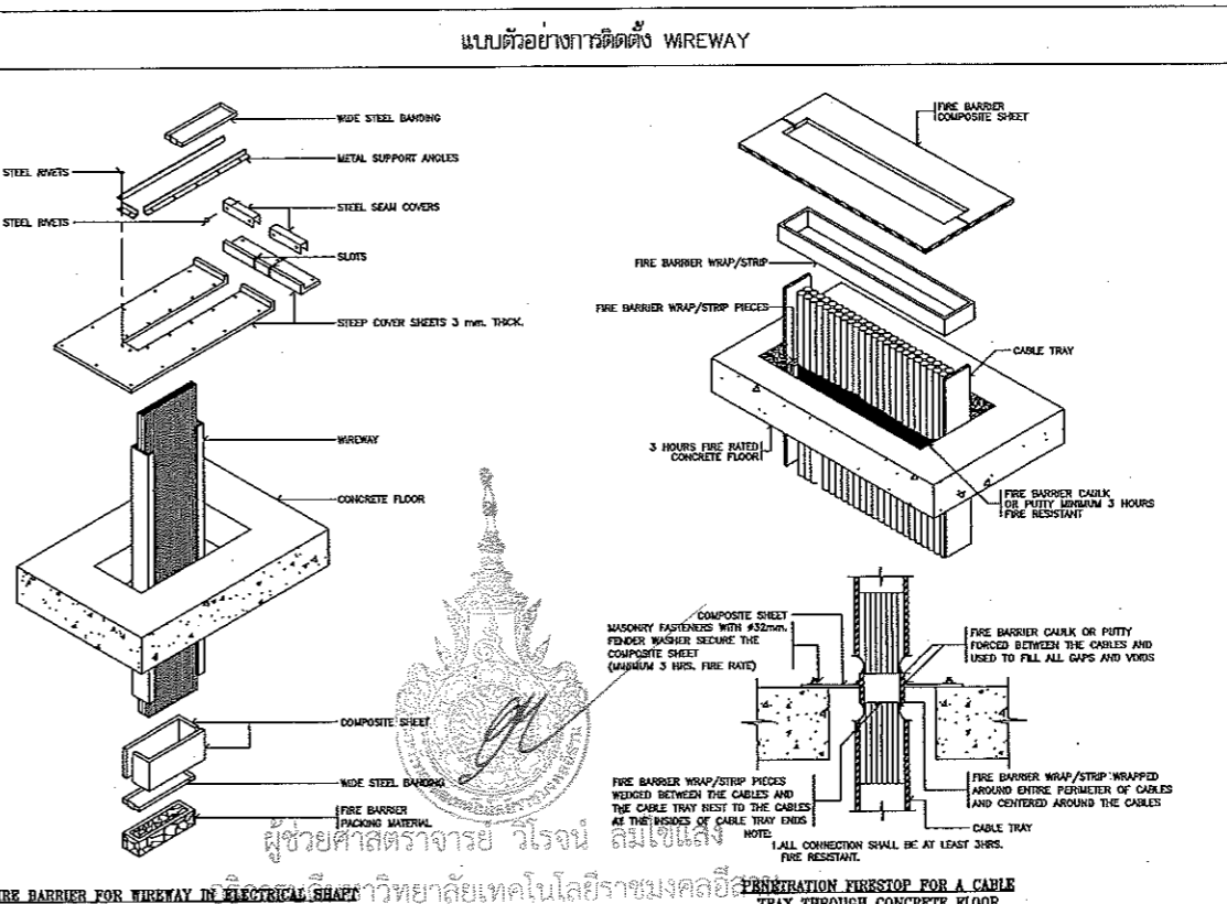
แบบตัวอย่างการติดตั้ง WAREWAY
