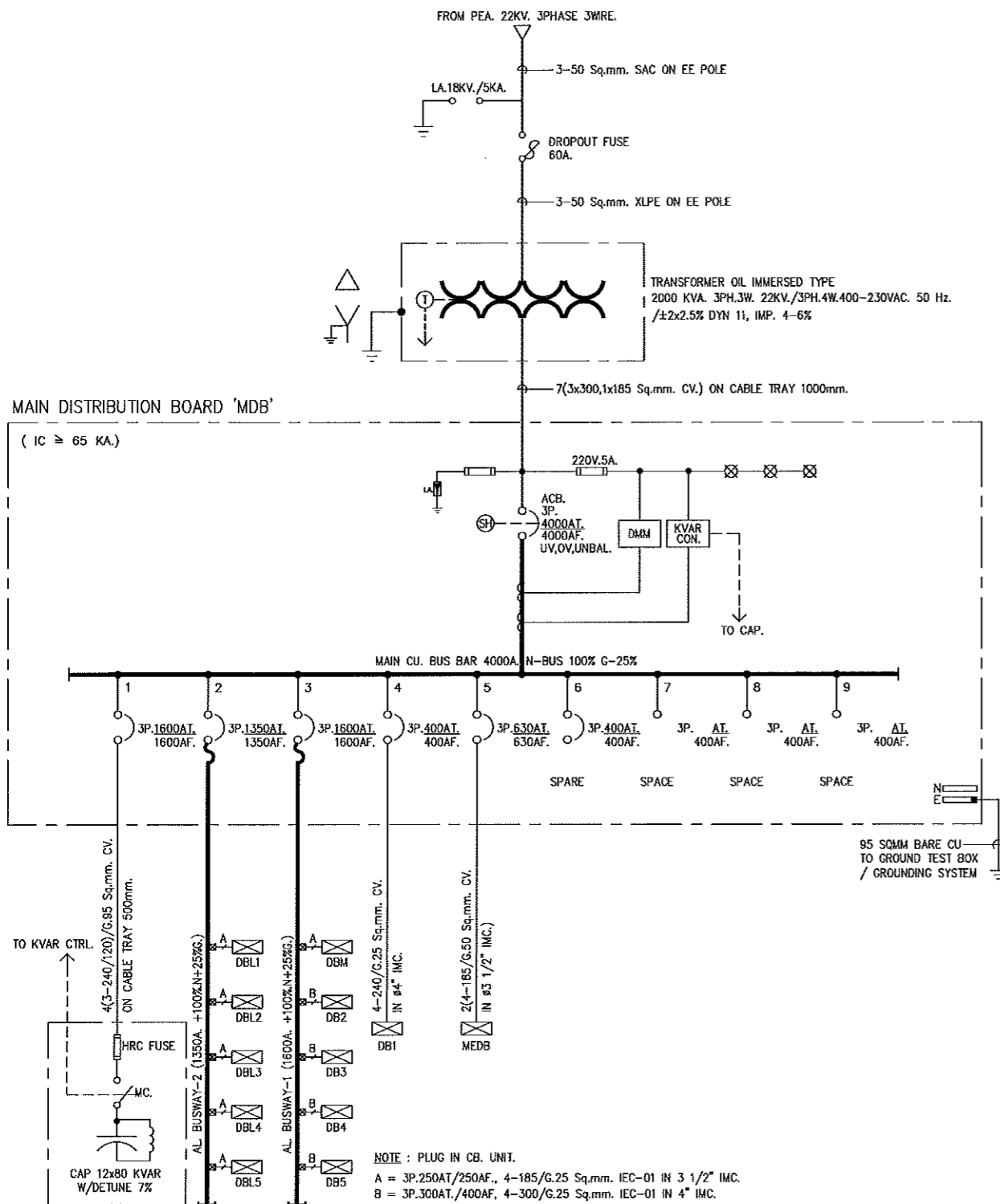
ไดอะแกรมระบบไฟฟ้า 1
