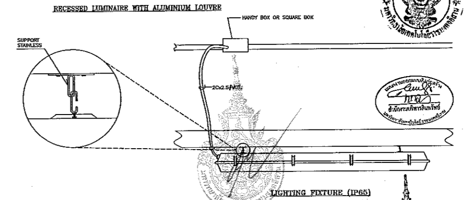
แบบตัวอย่างการติดตั้งโคมไฟ
