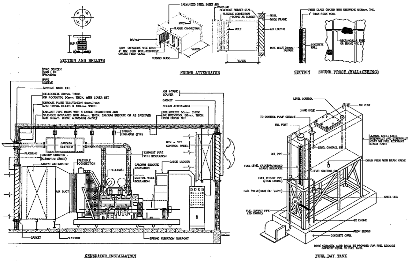
แบบตัวอย่างการติดตั้งเครื่องกำเนิดไฟฟ้าสำรอง
