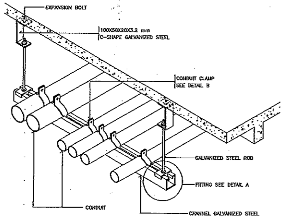
MULTIPLES CONDUIT SUPPORT
