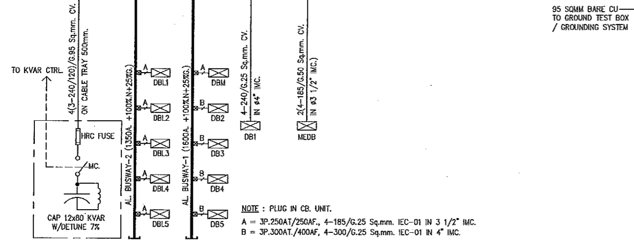
ไดอะแกรมระบบไฟฟ้า 1
