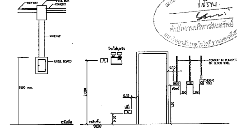
การติดตั้งตู้ควบคุมวงจรไฟฟ้า
