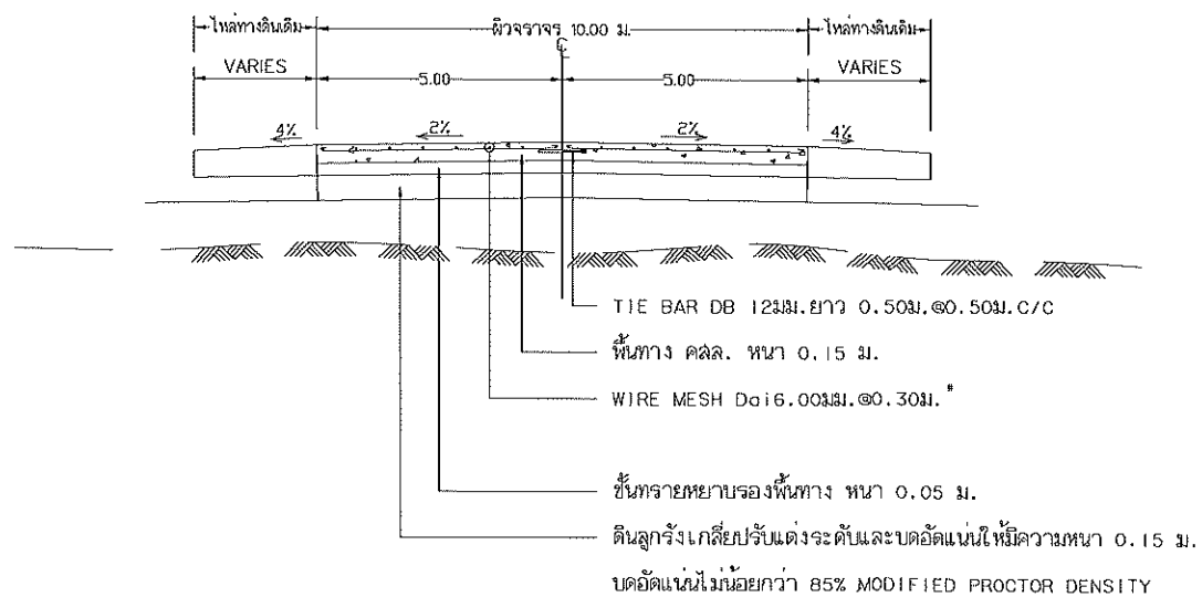
รูปตัดถนนผิวจราจรคอนกรีตเสริมเหล็ก กว้าง 10 เมตร
