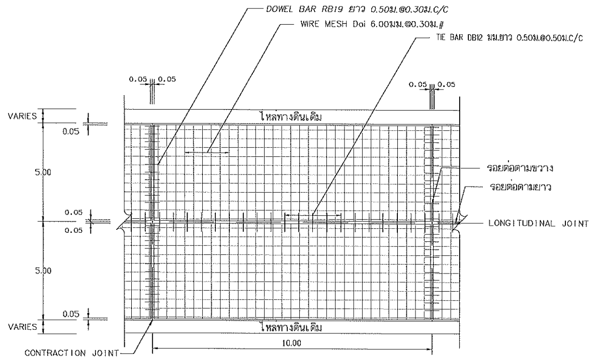
รูปแปลนผิวจราจรคอนกรีตเสริมเหล็ก กว้าง 10 เมตร
