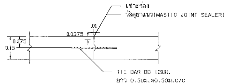
ขยายรอยต่อ LONGITUDINAL JOINT
